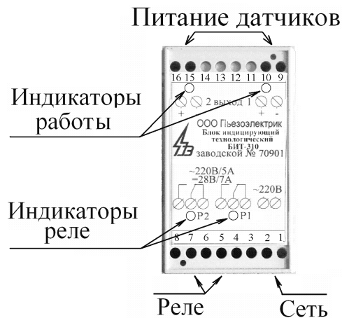
Рисунок 1 - Расположение клеммных колодок блока.
