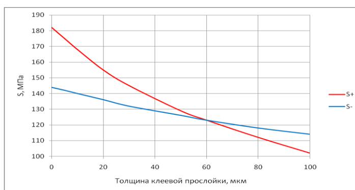
Рис. 4. Снижение максимальных растягивающих ( S^+ ) и сжимающих ( S^- ) напряжений в керамике за счет клеевых прослоек
