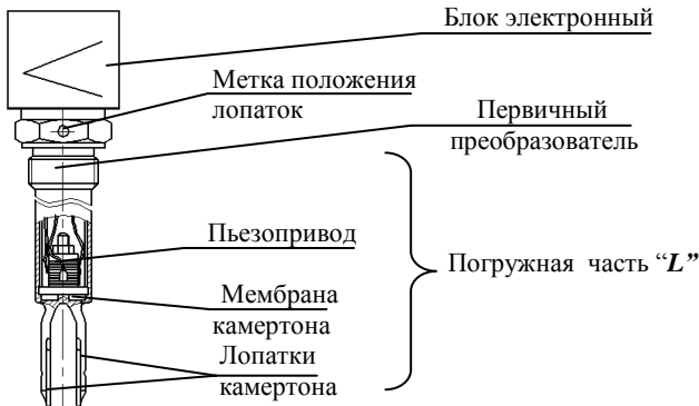
Рисунок 2 – Схема СУ
