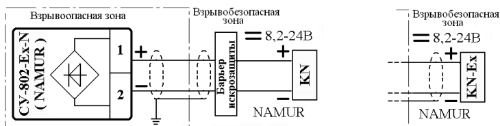
- а - с барьером искрозащиты
