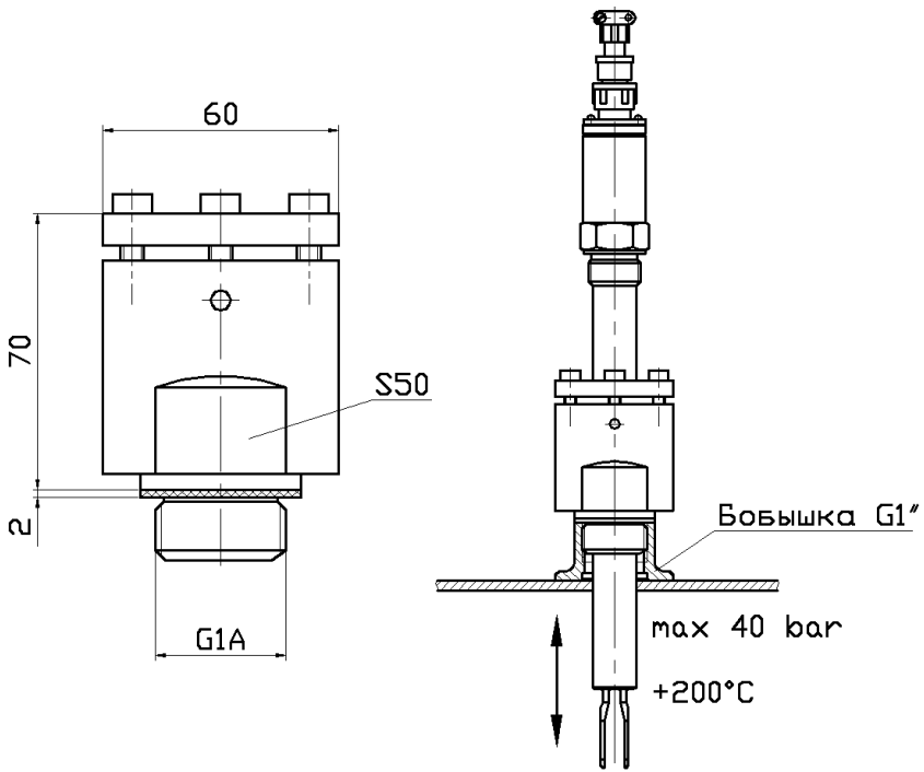
Рисунок А.3 – Втулка передвижная и установка СУ
