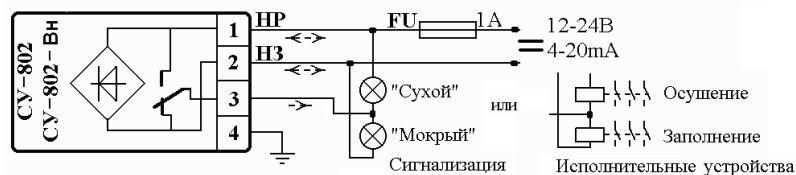
СУ обычного и взрывозащищенного Вн-Д исполнений
