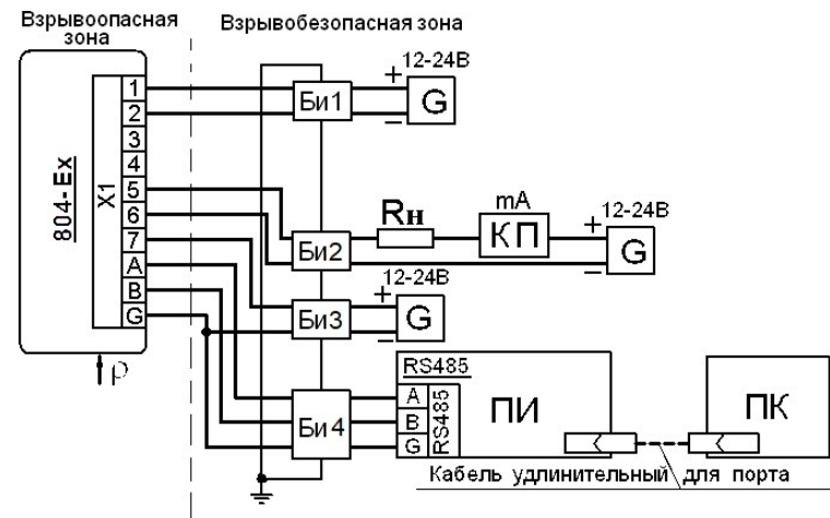
Рисунок В.3 - Схема подсоединения внешних электрических цепей плотномеров 804-Ex
