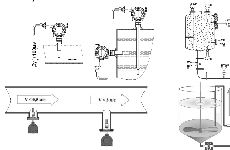
Рисунок 2 – Варианты монтажа плотномеров
