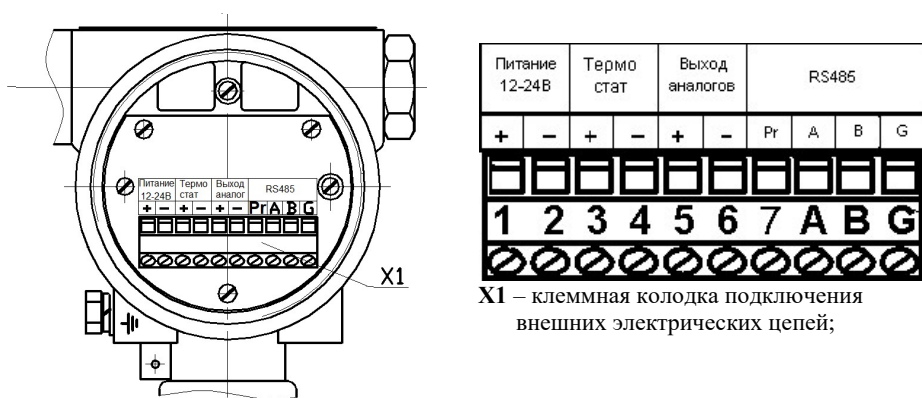
Рисунок В.1 – Вид на монтажную плату
